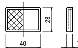
反射板詳細図
