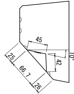
A-A 矢視詳細図
