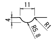
凹模様部詳細図
