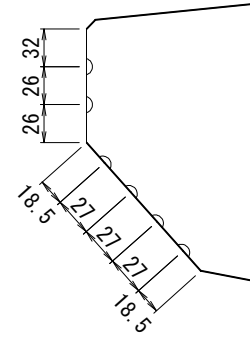
B-B 矢視詳細図
