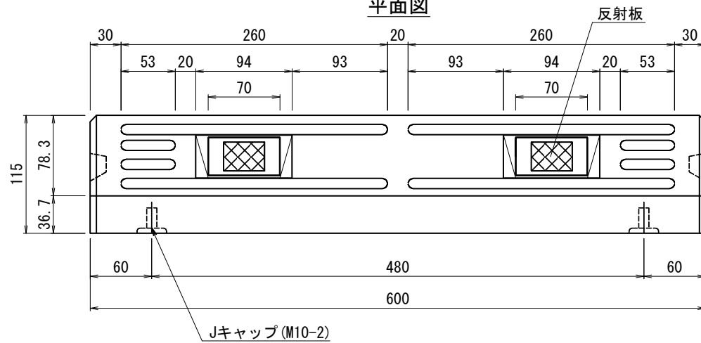
反射板取付プレート詳細図
