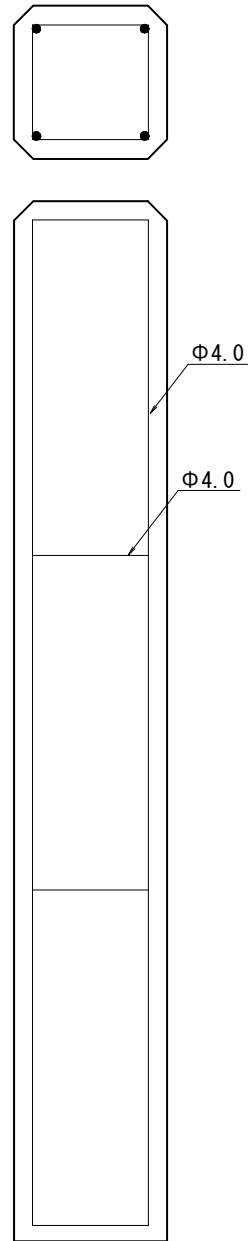
配筋図
